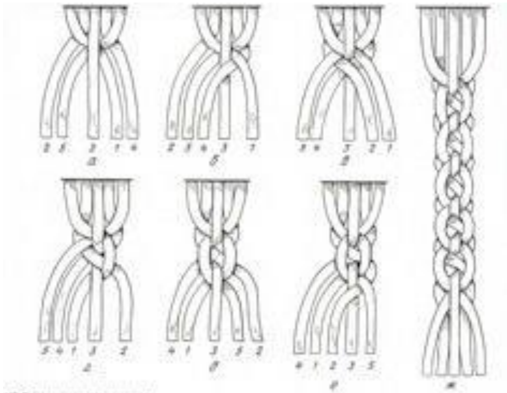
188. Пошаговое описание плетения каната из пяти прядей (a-g)
