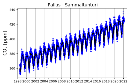
Bild 1: Koncentrationen av koldioxid i atmosfären i Sammaltunturi, Pallas, Lapland. Enheten (ppm = parts per million) betyder en miljondel av molekylerna i atmosfären. Källa: Meteorologiska institutet
