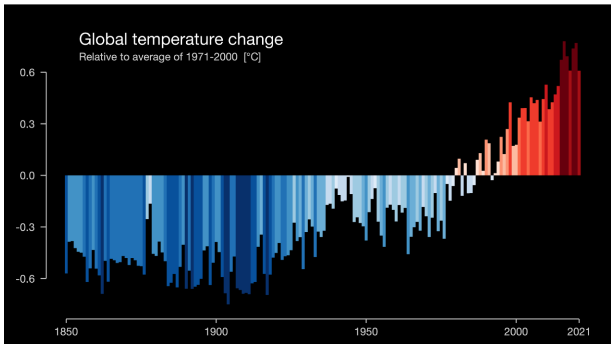
Bild 2: Jordens medeltemperatur, förändringen i grader jämfört med medelvärdet av åren 1971-2000. Källa: Ed Hawkins, University of Reading, https://showyourstripes.info/c/globe
