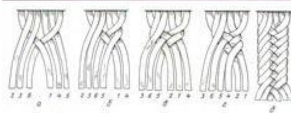
189. Описание плетения каната из 5 прядей в технике «косичка» (a-e)
